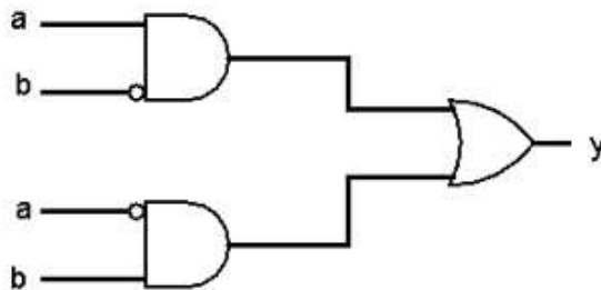
Figura 5.9: Função com duas variáveis
